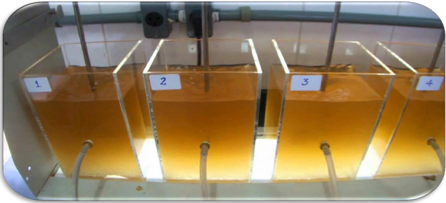
Figura V I Aparelho utilizado para realização dos ensaios de tratabilidade
